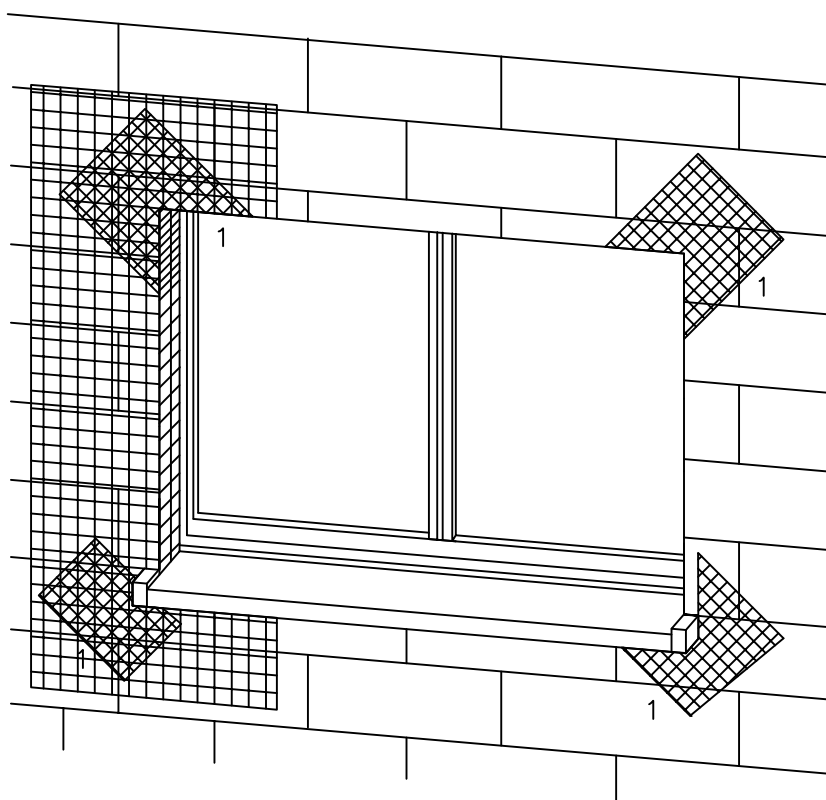
1 Zbrojenie diagonalne; Paski siatki (min. 20x30cm)
